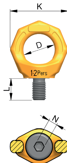
Abb. 3: Maßzeichnung PSA VRS für 1-2 Personen
