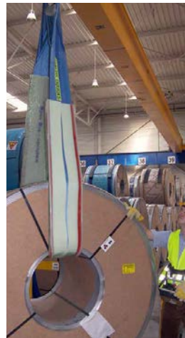
Clipschlauch-SC für SpanSet-Schwerlast-Powerband CS nach Abbildung 1
