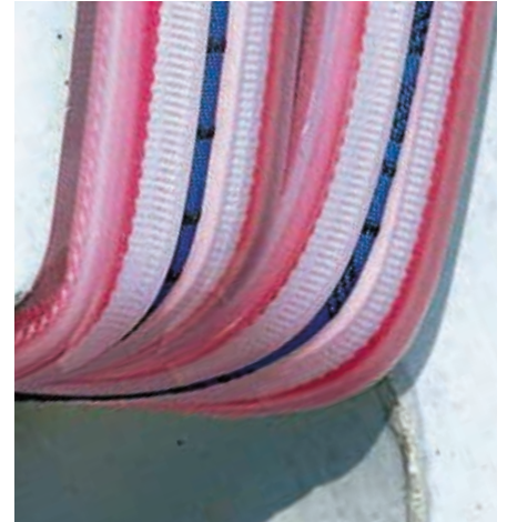
Clipschlauch-SC für SpanSet-SupraPlus- und MagnumPlus-Rundschnle nach Abbildung 3 oder 5
