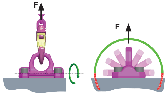
Abb. 3: Wendevorgänge in Klapprichtung
