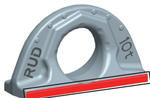
Abb. 2: Bereich des Schweißnahtübergangs
